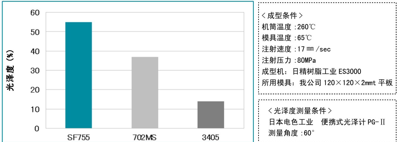
图4 - 1 SF755与常规等级的光泽度比较
