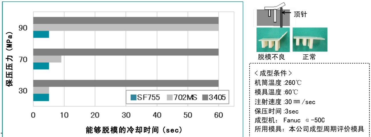
图2 - 1 SF755与常规等级的脱模性比较
