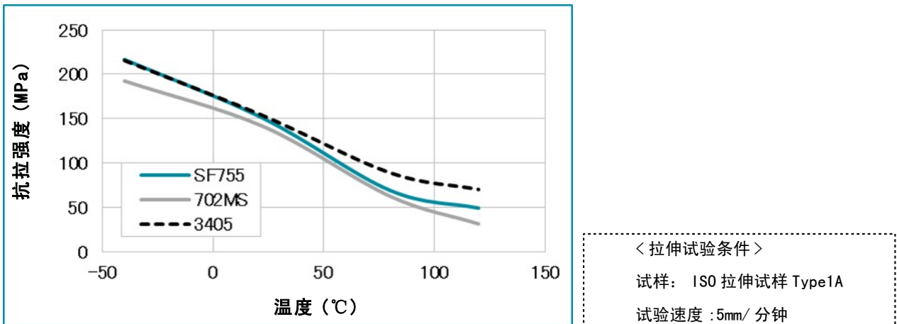
图6 - 1 SF755与常规等级的拉伸强度-温度关系比较
