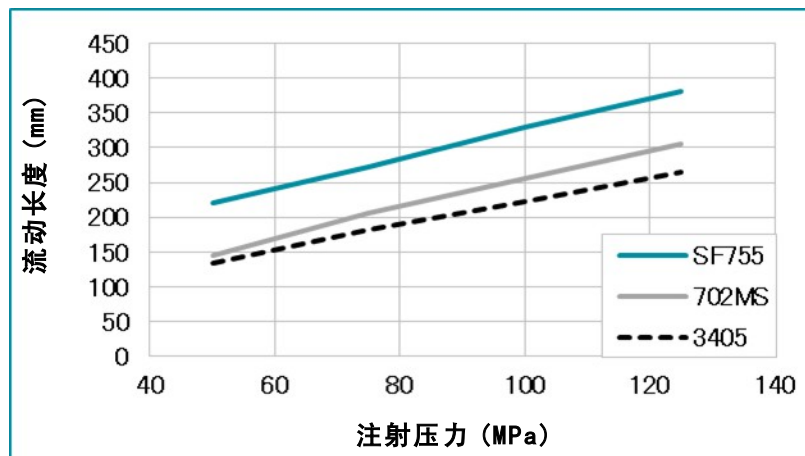
图3-1 棒流动长
