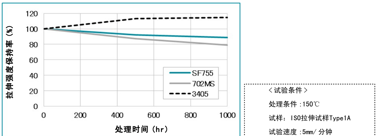
图5 - 1 SF755与常规等级的耐热性比较
