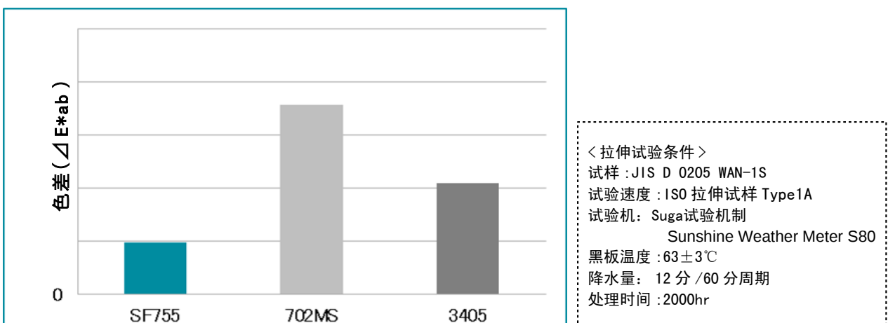
图7 - 1 SF755与常规等级的耐候性比较
