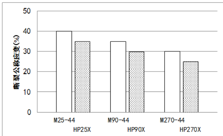
图 1-2 HP-X系列与普通等级的拉伸断裂公称应变的比较 (ISO 527, 23℃)
