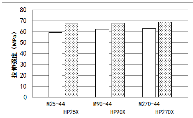
图 1-1 HP-X系列与普通等级的拉伸强度的比较 (ISO 527, 23℃)
